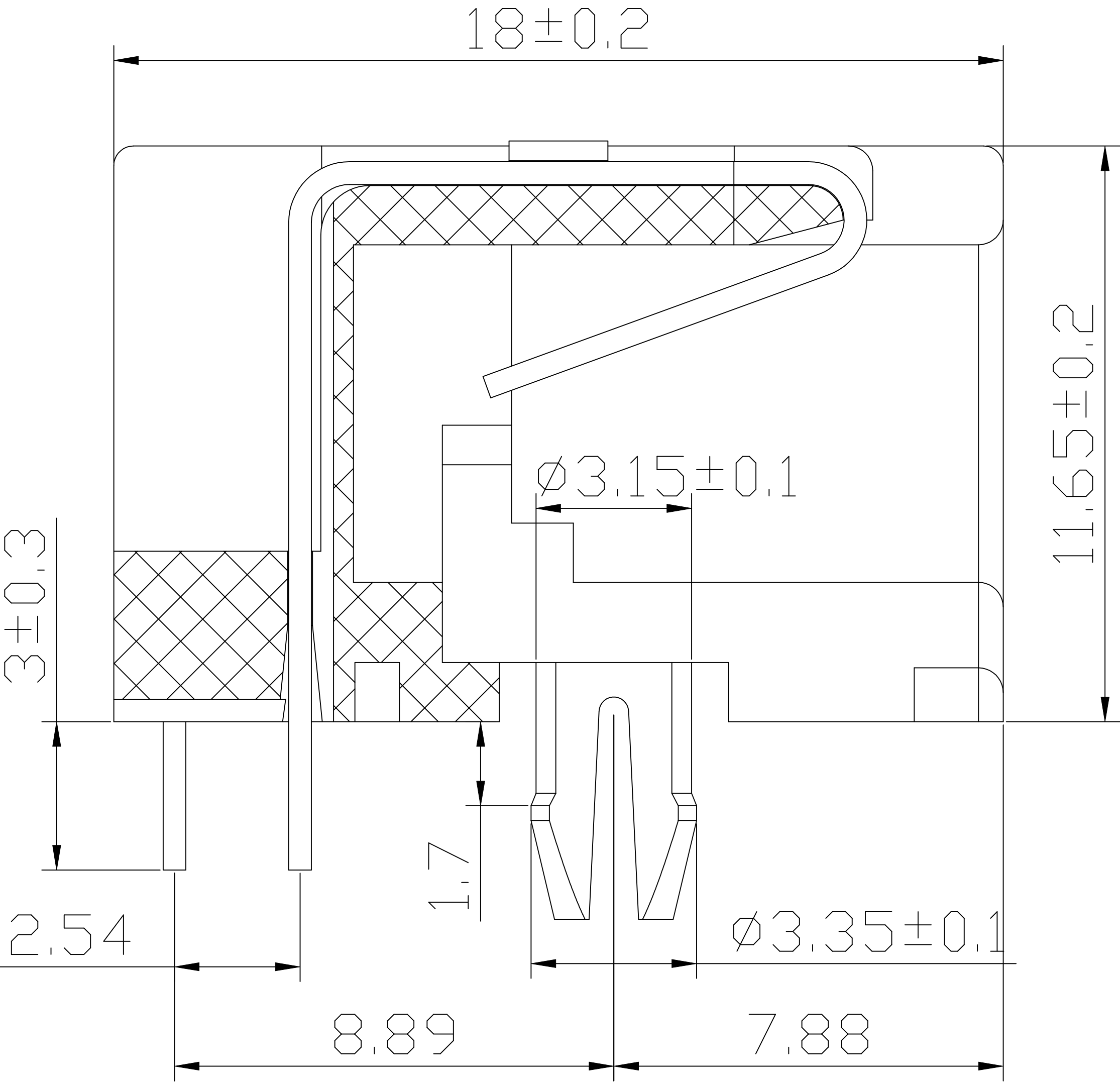
SECTION A-A
