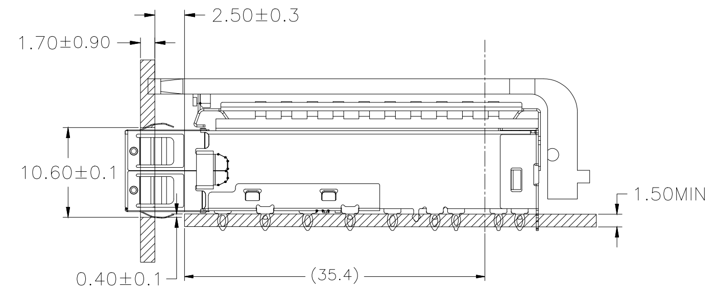
SECTION A-A
